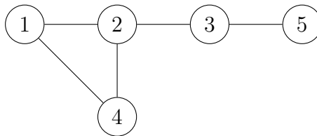
Figure 1: Exemple d'un graphe de Barabási-Albert montrant l'attachement préférentiel.
